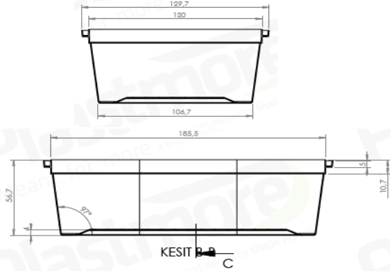
Tub / Kutu
