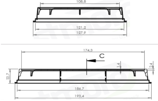
Lid / Kapak
